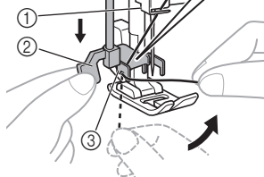
① Suport pentru ac ② Pârghie dispozitiv de înfilare ac ③ Conducător de fir
