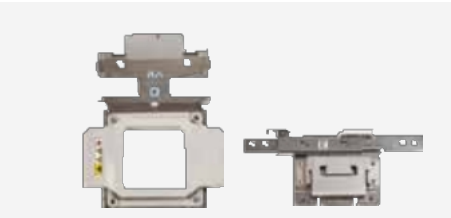
PRMFA50 Gherghef magnetic și braț 50 x 50 mm Această ramă vă permite să brodați țesături fără a lăsa urme de cusături, în special în cazul țesăturilor predispuse la acest lucru. Braț E inclus. Dacă aveți deja acest braț, vă rugăm să alegeți numai rama magnetică PRMF50.
