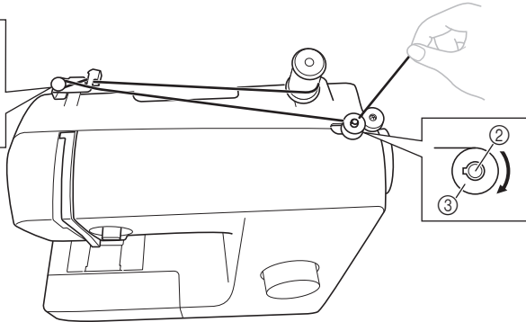
1 Disc de pretensionare 2 Axul bobinatorului 3 Bobină
