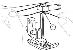
① Conducătorul de fir de pe tija de fixare a acului
